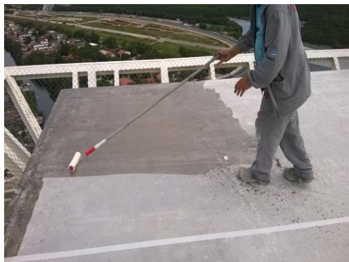
APLICAÇÃO DE PRIMER + REVESTIMENTO ARGAMASSADO
