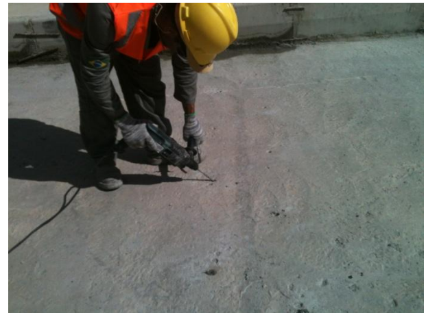
FURAÇÃO - INSTALAÇÃO DOS BICOS DE PERFURAÇÃO
