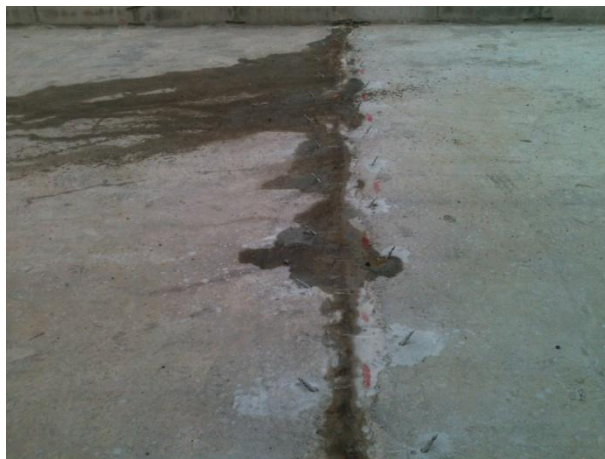
BICOS DE PERFURAÇÃO INSTALADOS
