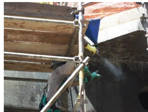
PREPARAÇÃO DO SUBSTARTO (ESTUCAMENTO COM AREIA WR)
