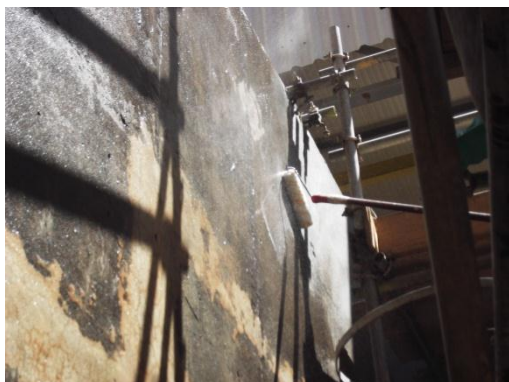
PREPARAÇÃO DO SUBSTARTO (APLICAÇÃO DE PRIMER)
