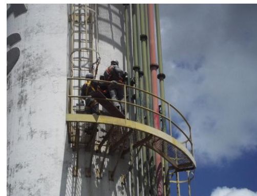
INSTALAÇÃO DE EQUIPAMENTOS (GHUINCHO E MÃO FRANCESA)
